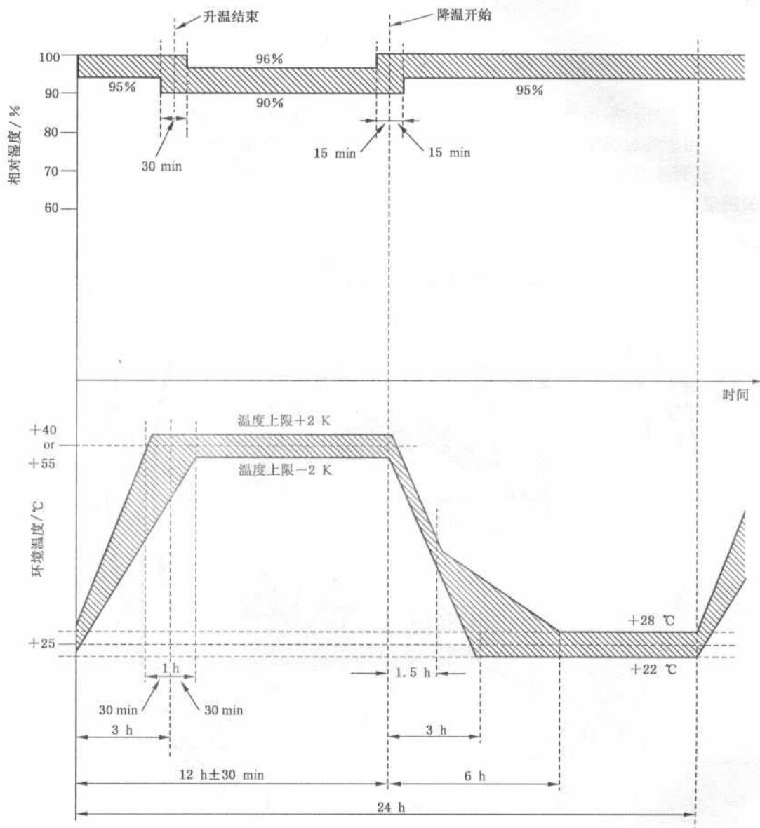
图 1 试验 Db 试验周期
